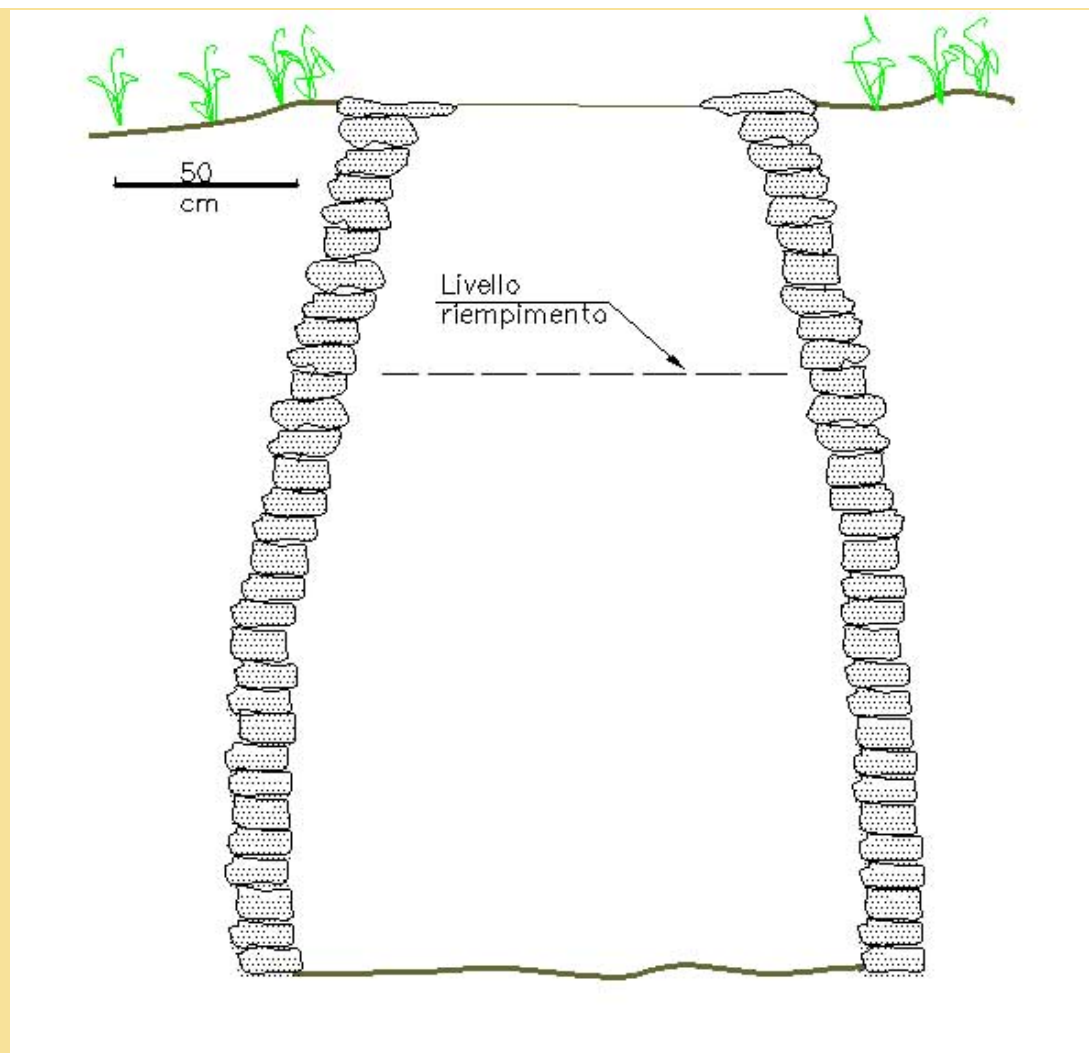
Figura 2) Schizzo ricostruente la struttura di una tipica loera di Polaveno
