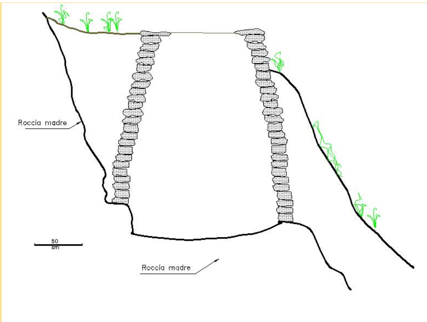
Figura 3) Rilievo di una tipica loera di versante di Polavento
